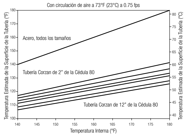
Figura 7 Temperatura Estimada de la Superficie de la Tubería contra la Temperatura Interna del Fluido
