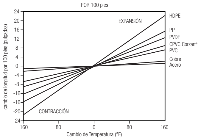
Figura 3 Expansión térmica de materiales de tubería
