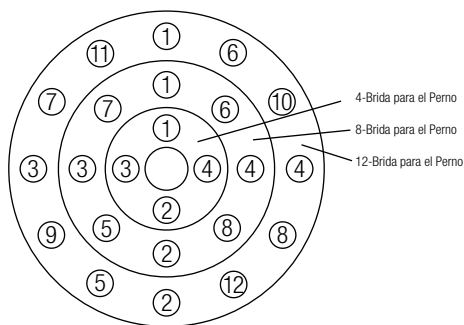
Figura 5 Patrones para la Sujeción del Tornillo de la Brida
