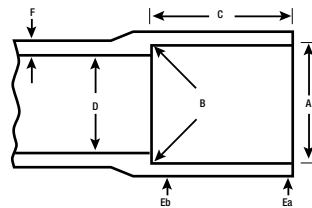
Figura 1 Dimensiones del Adaptador Cónico* para las Conexiones Corzan Cédula 80 de acuerdo con ASTM F439
