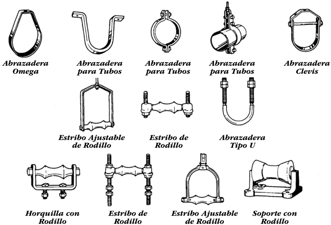
Figura 6 Sujetadores, Abrazaderas y Soportes de Tubería
